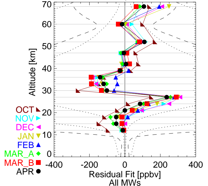
O3 REC analysis - Altitude
