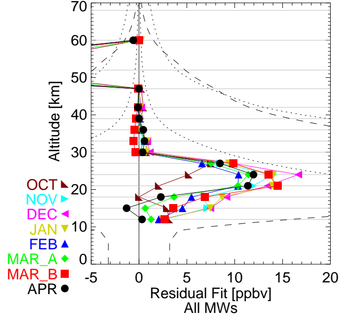
O3 REC analysis - Altitude
