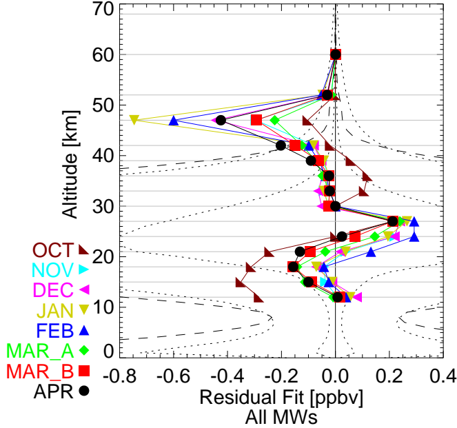
NO2 REC analysis - Altitude
